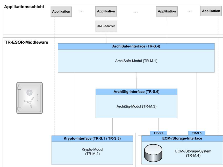
Abbildung 4: TR-ESOR Referenzarchitektur
