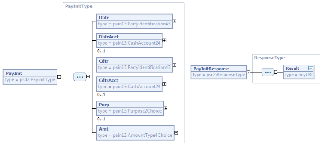
Abb. 2: Schnittstelle zum Auslösen eines Zahlungsvorgangs (Art. 66)
