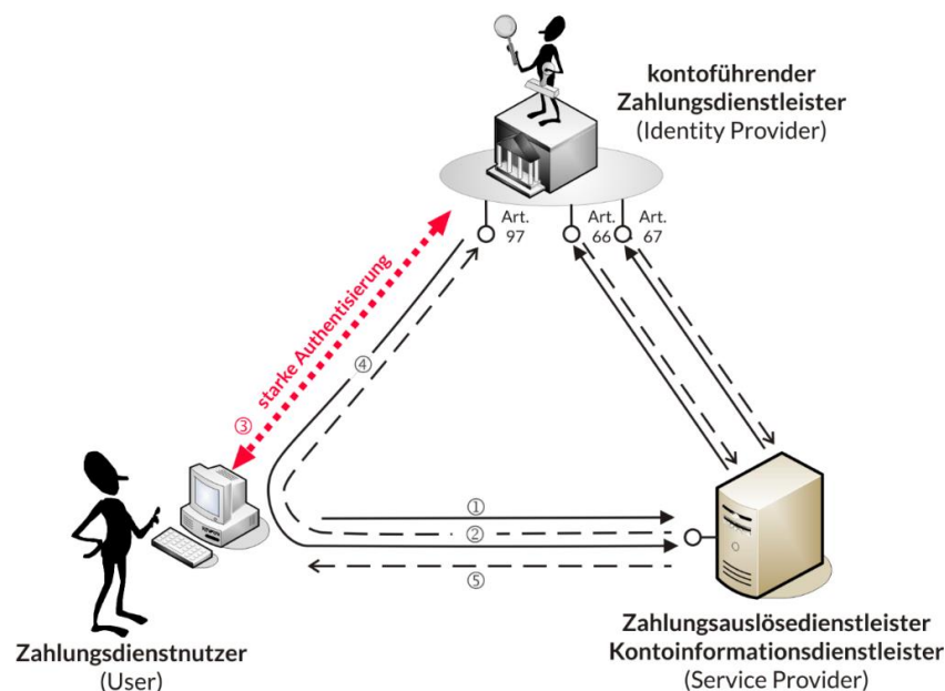
Abb. 1: Zusammenwirken der Zahlungsdienstleister gemäß PSD2-Richtlinie
